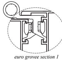
euro groove section 1
