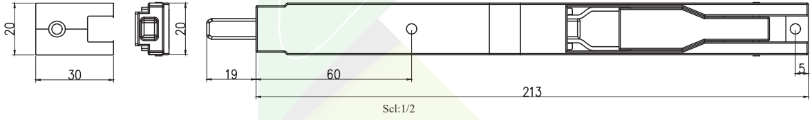
KRC-7002 Isı yalıtım Zamak sürgü Zamak lever bolt
