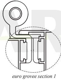
KRC-3309 Karaca kapı-pencere menteşesi Karaca Window-door hinge Euro Section-kanal 1
