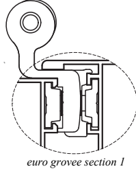
euro groove section 1
