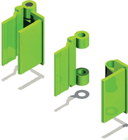
KRC-3002 Aldoks geçme menteşe Aldoks slip in hinge
