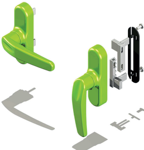
KRC-1703 Çift maçalı eksenel kol Double plate window handle
