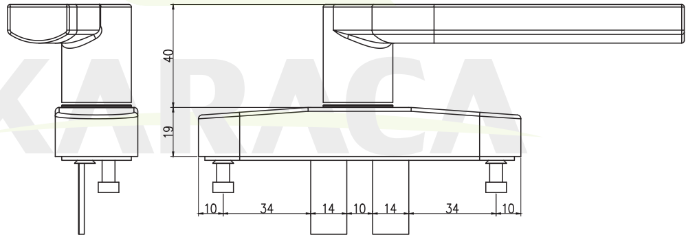
KRC-1705 Çift maçalı cephe kolu Hidden sash window handle double plate
