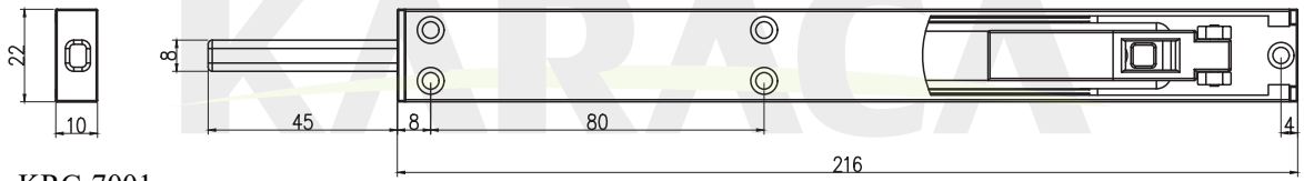
KRC-7001 C-60 Atlamalı uzun sürgü Lever bolt (long)
