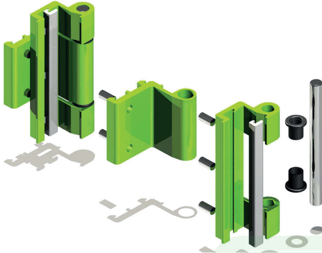
KRC-3300 Saray 94 seri pencere-kapı menteşe Window-door hinge
