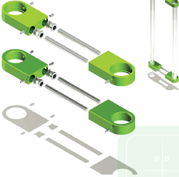
KRC-1157 Akbank kol ve aparatı Tube pull handle
