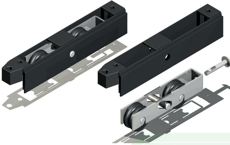
KRC-7550 Çift makaralı ayarlı rulman Double adjustable roller
