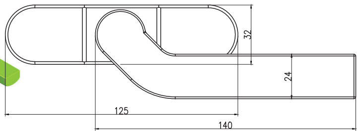
KRC-1705 Çift maçalı cephe kolu Hidden sash window handle double plate
